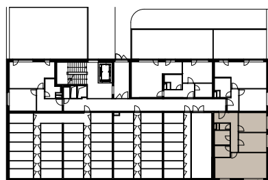
plán podlaží
